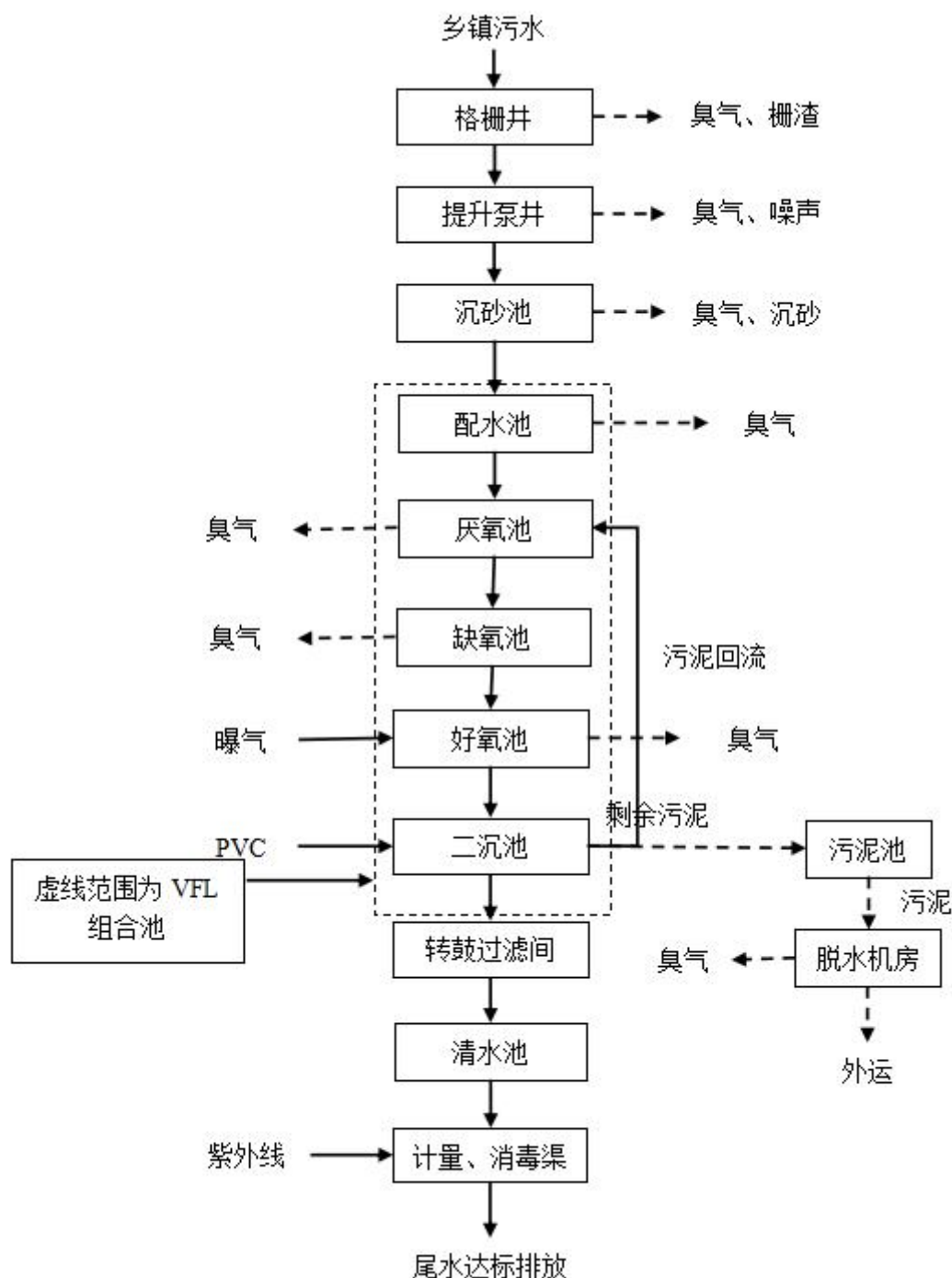
图 2.2-1 大忠桥镇污水处理厂工艺流程及产污环节图
