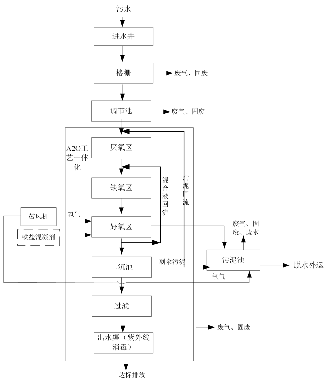
图 2.2-1 茅竹镇污水处理厂工艺流程及产污环节图
